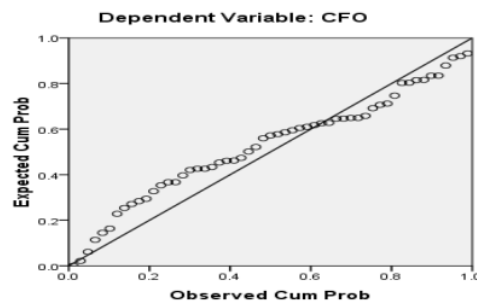
Gambar 3. Hasil Uji Normalitas
