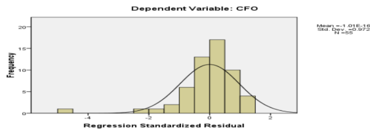
Gambar 2. Histogram Uji Normalitas
