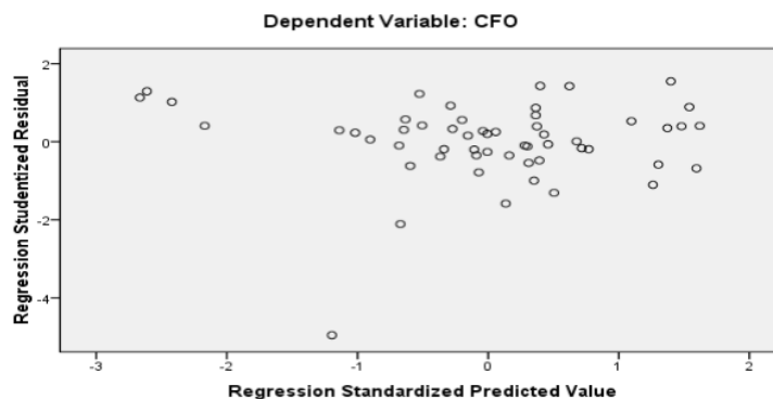
Gambar 1. Grafik Scatterplot untuk Uji Heteroskedastisitas
